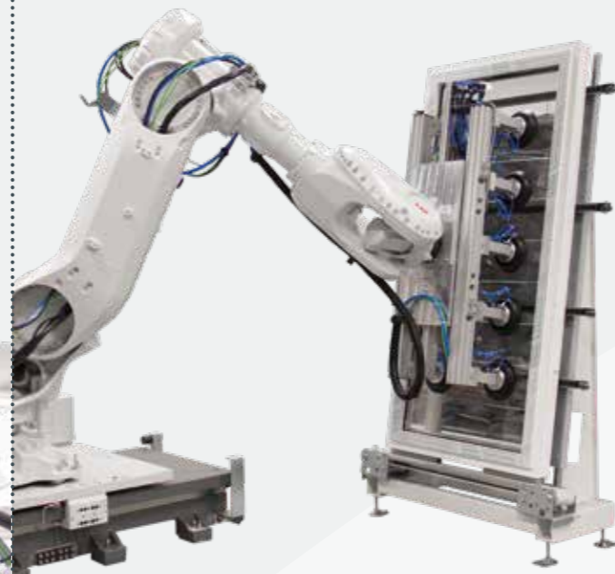
automatisches Einlegen der Glasscheiben in fertige Elemente panels placed automatically in the finished elements
