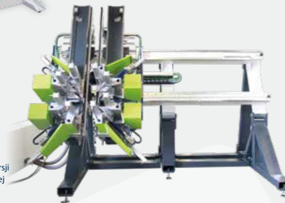
Формирователь уплотнителя Formery uszczelki
