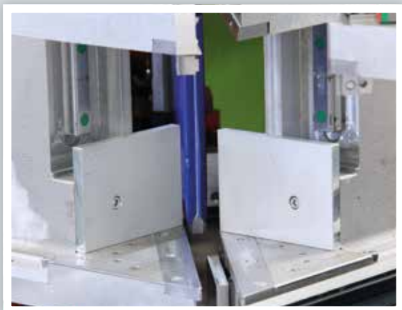
Смена цулаг без инструмента System wymiany podpór profilowych bez narzędzi
