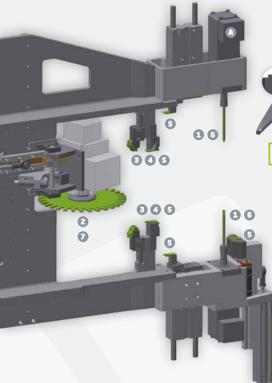
verschiedene Messervarianten different blade versions
